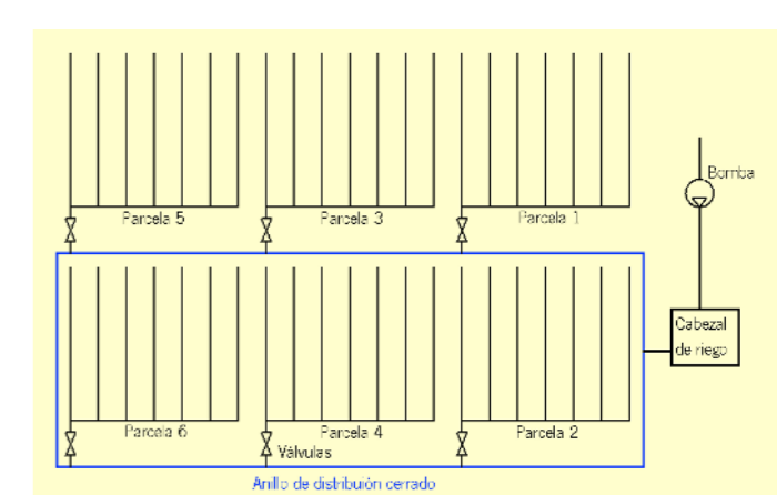
Sistema de distribución en anillo cerrado.
